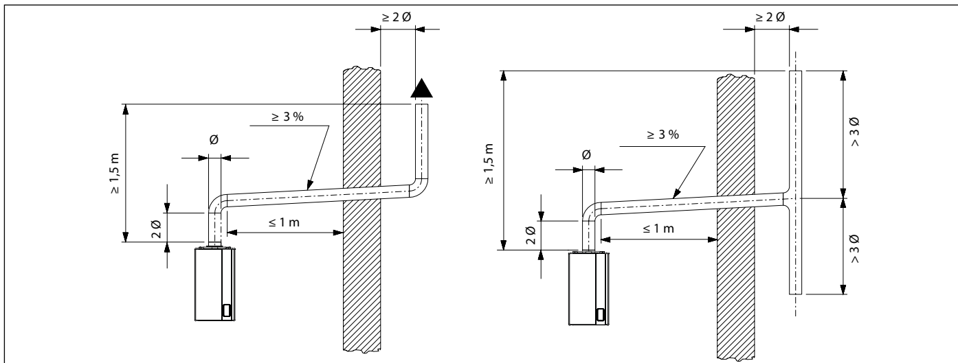
6. ábra – Nyílt égésterű modell füstgáz elvezetése kéménybe
