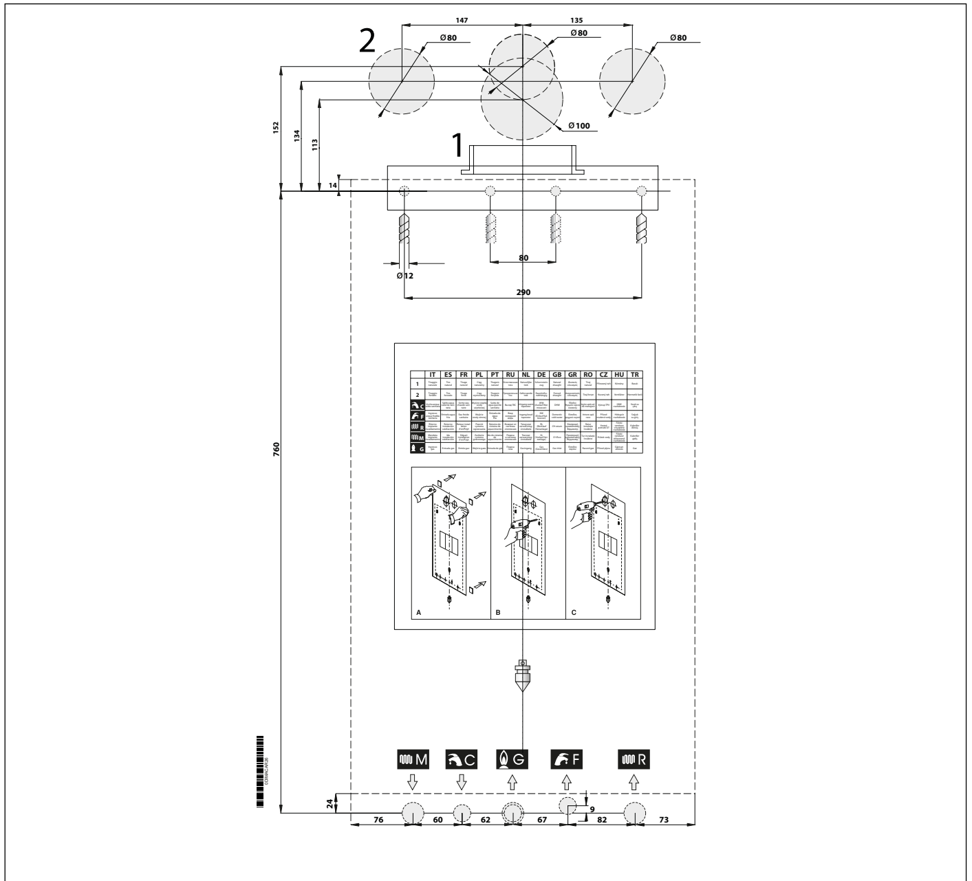
5. ábra – Rögzítősablon
