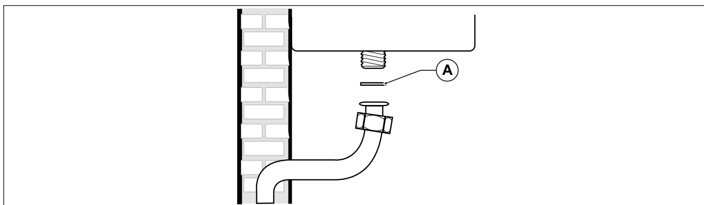
8. ábra – Csatlakozás a gázvezetékhez
